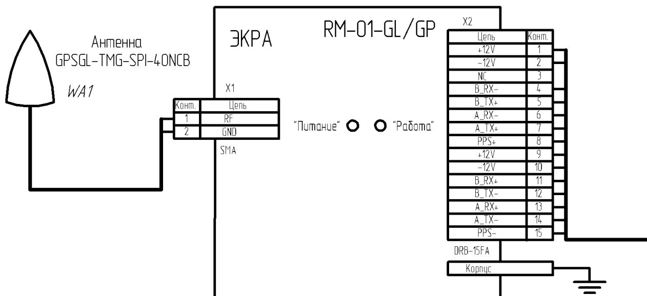
Рисунок 17 – Схема включения приемника RM-01-GL/GP
