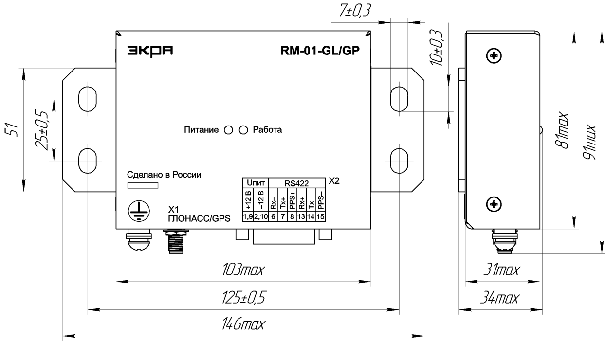
Рисунок 4 – Общий вид приемника RM-01-GL/GP-01
