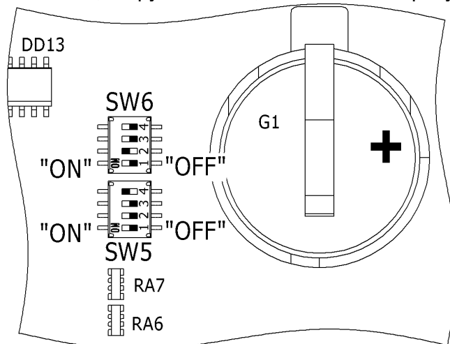
Рисунок 15 – Переключатели SW5, SW6
