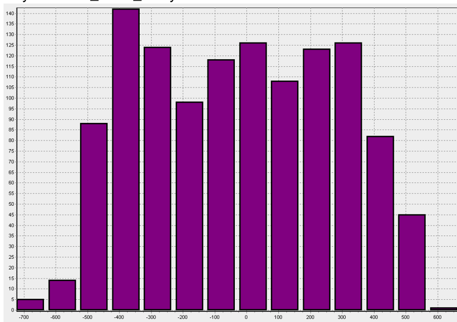
Рисунок 21 – Гистограмма распределения абсолютной ошибки синхронизации (нс) в режиме E2E GrandMaster – E2E Slave (между PTP устройствами включен pop - PTP свитч MOXA EDS-408A-MM-ST)
