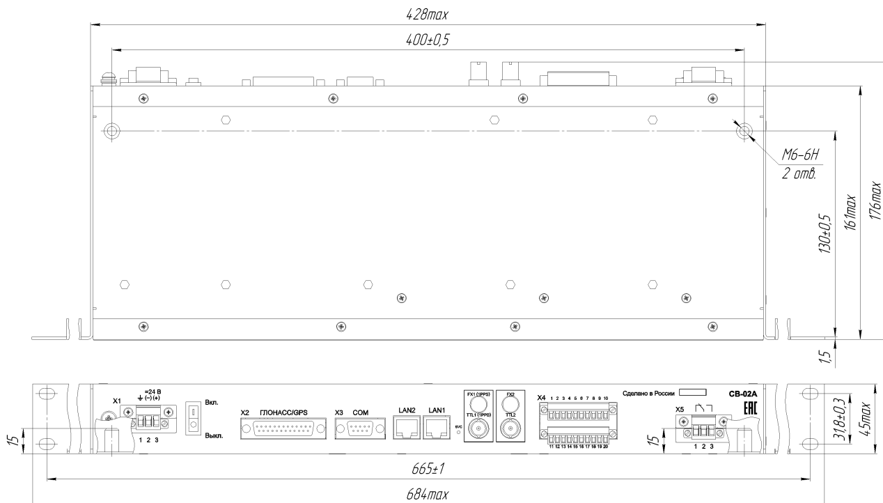
Рисунок 2 – Общий вид устройства СВ-02А (исп. -02)
