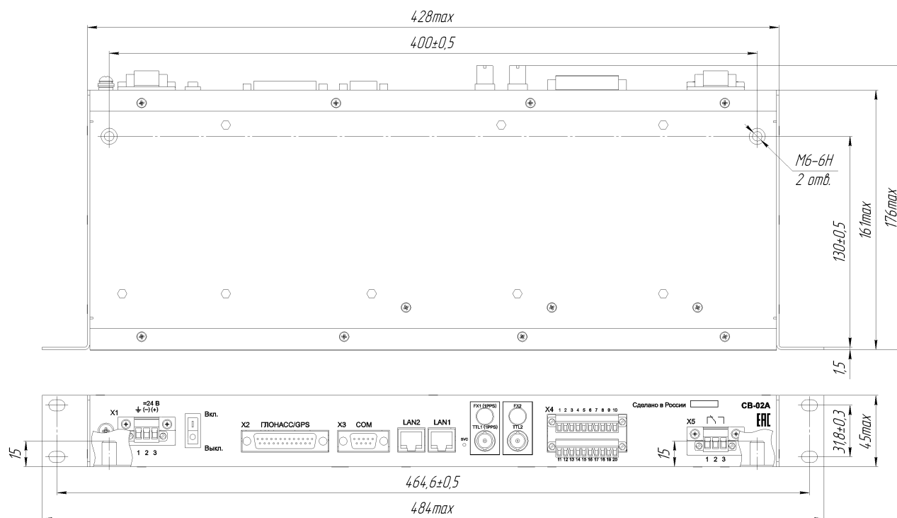
Рисунок 1 – Общий вид устройства СВ-02А (без исп.)
