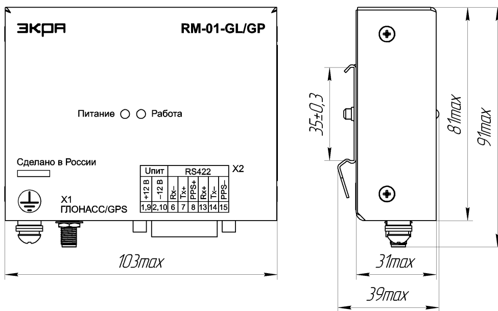
Рисунок 3 – Общий вид приемника RM-01-GL/GP
