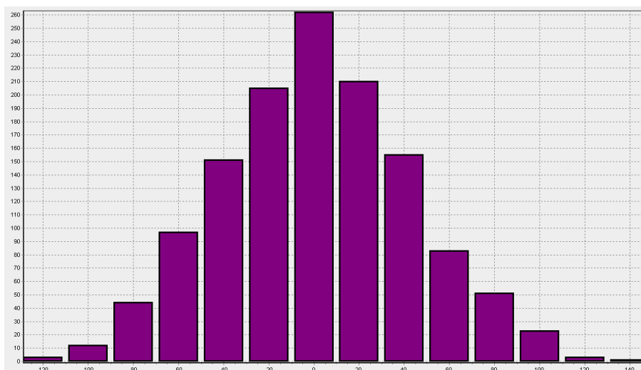
Рисунок 20 – Гистограмма распределения абсолютной ошибки синхронизации (нс) в режиме E2E GrandMaster – E2E Slave OC (между PTP устройствами включены «прозрачные» часы на базе RSG2288NC)
